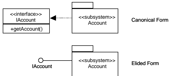
Fig. 2. UML component
